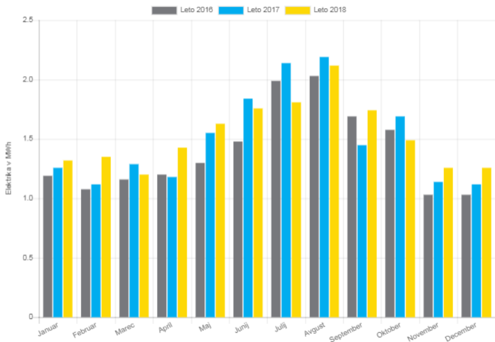
Poraba električne energije za vsa merilna mesta za objekt Planinski dom na Sviščakih
